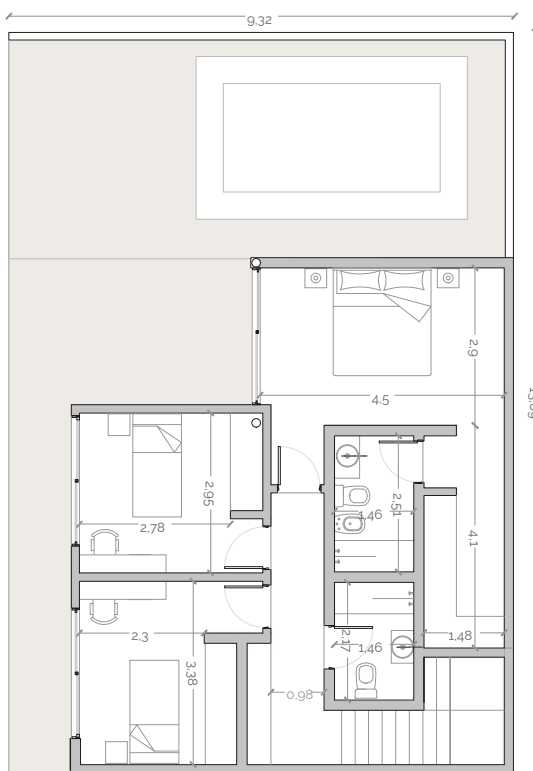
PLANTA ALTA
