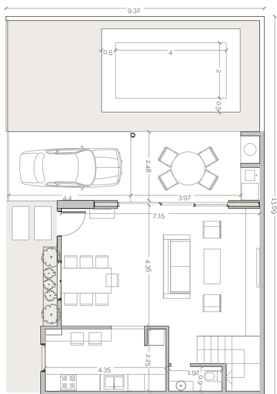
PLANTA BAJA
