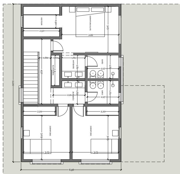
PLANTA ALTA
