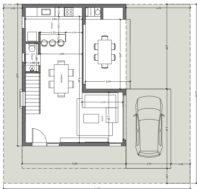
PLANTA BAJA
