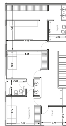
PLANTA ALTA
