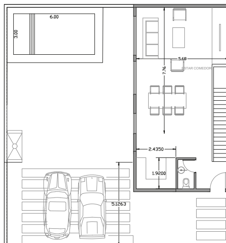
PLANTA BAJA
