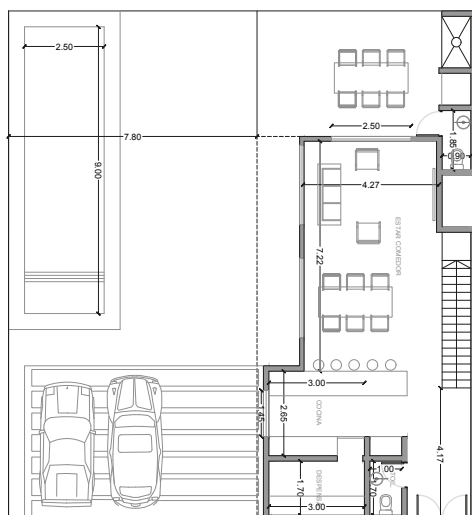
PLANTA BAJA
